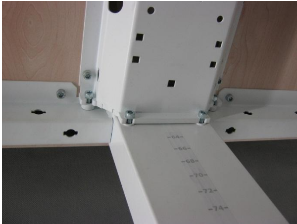
Figuur 7: Beproefd exemplaar 12.0866-1 van Voortman Hi Tee wangen bureautafel, slingerverstelbaar- bevestiging traverse aan poot
